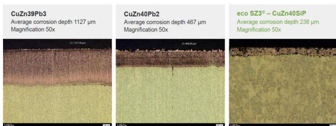
Figure 5-5: ECO SZ3 corrosion behaviour (EN ISO 6509)(CuCl 2 / 75 °C / 24 h)
